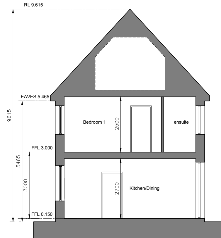
Section A-A
